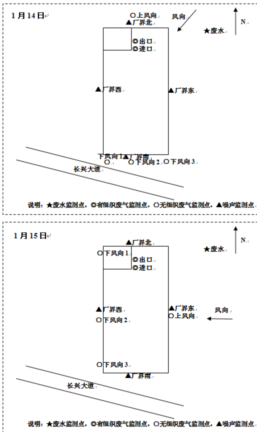
图 7-1 项目监测点位示意图
