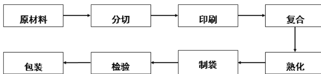
图 3.6-2 萧山瑛源彩印软包装厂工艺流程图
