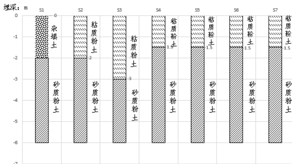
图 6.1-1 土层剖面图
