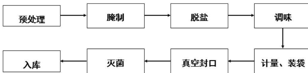
图 3.6-6 义蓬乐河桥菜厂工艺流程图
