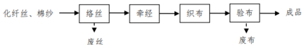
图 3.6-4 强顺化纤工艺流程图
